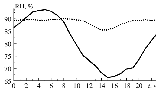
Рис. 7. Среднемесячный суточный ход относительной влажности; --- – январь, — июнь (1996)
