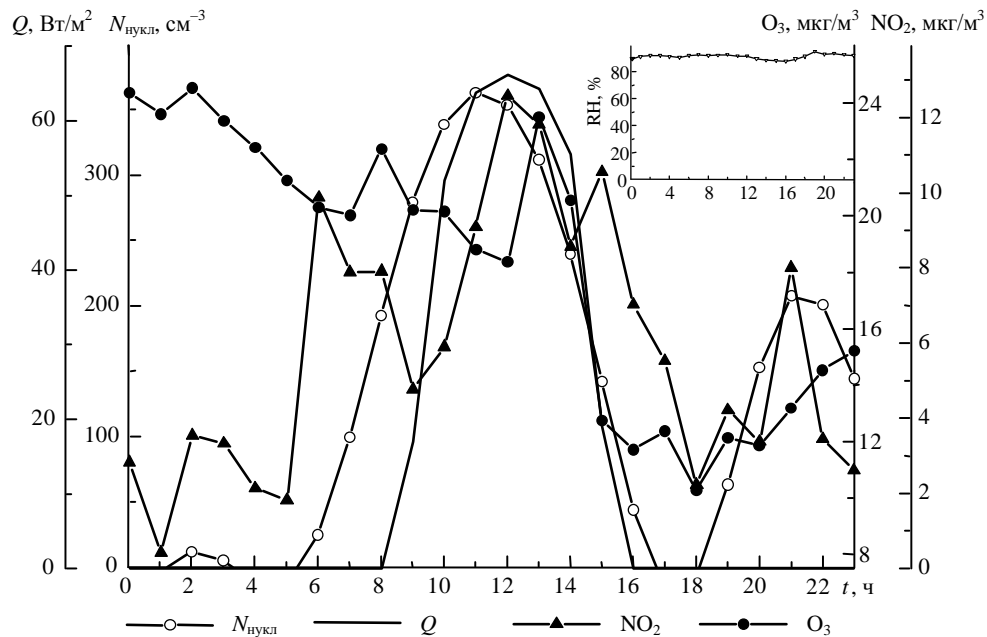
Рис. 8. Суточный ход счетной концентрации аэрозоля d = 0,003 - 0,008 мкм ( N ), озона ( O_3 ), двуокиси азота ( NO_2 ), интенсивности солнечной радиации ( Q ) и относительной влажности ( RH ); 17 декабря 1998 г.
