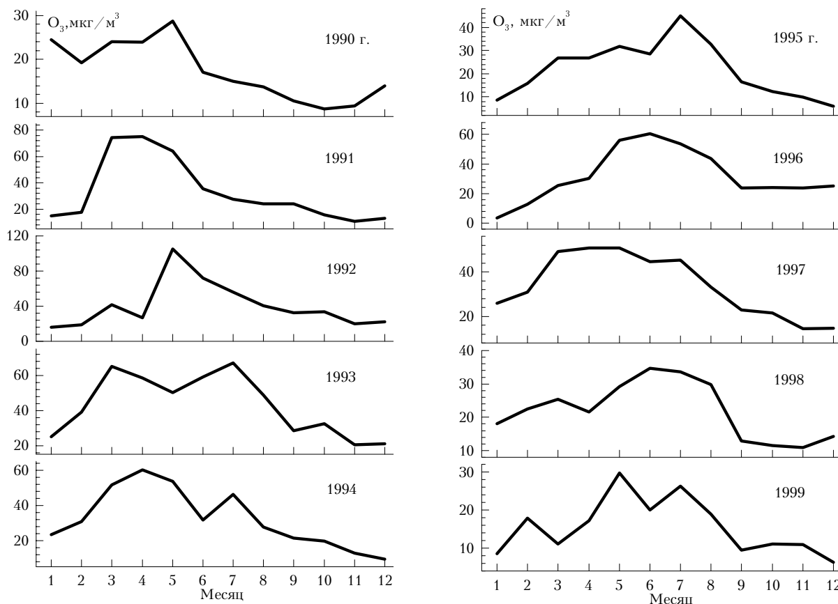
Рис. 2. Сезонный ход концентрации озона для Томска в различные годы
