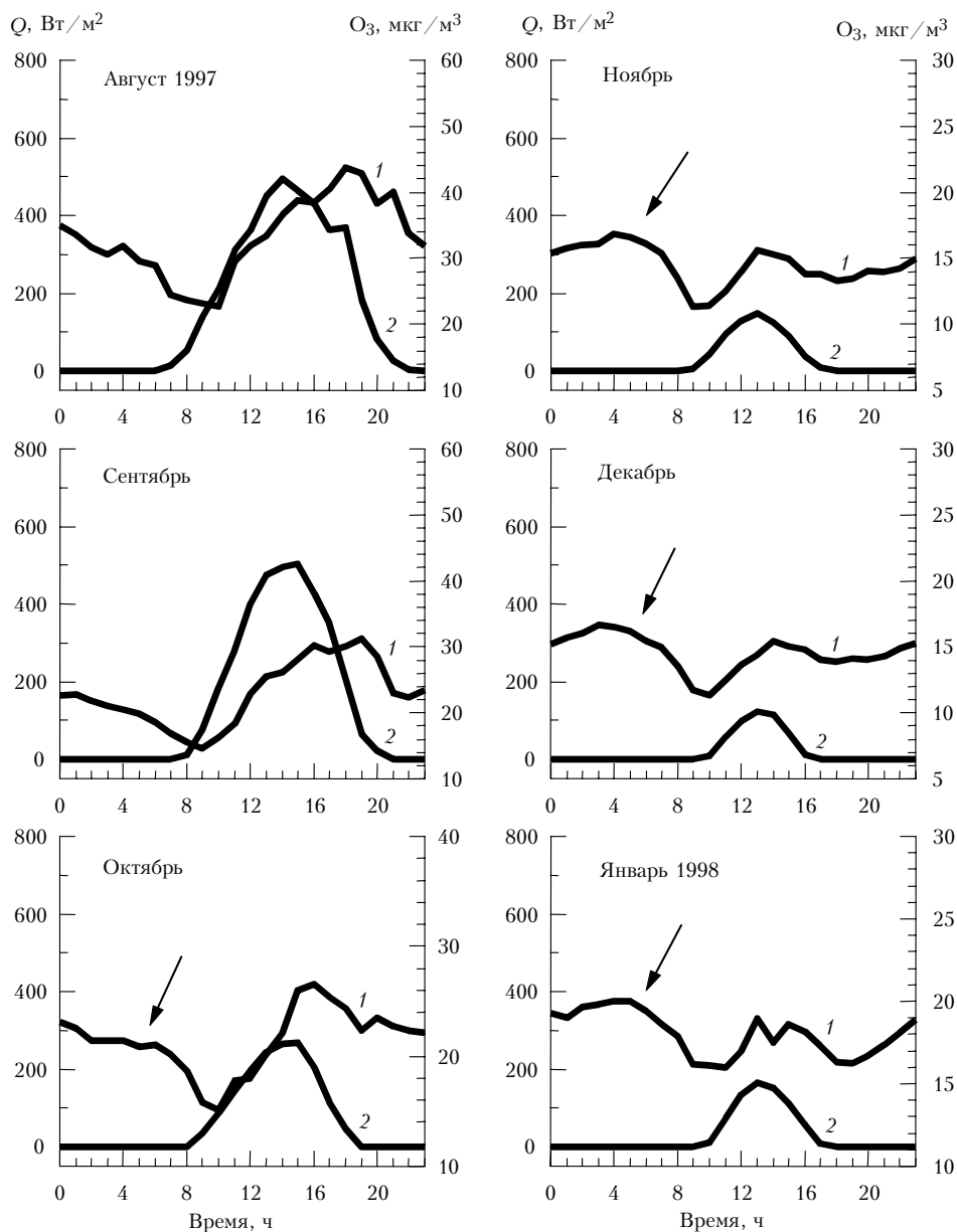
Рис. 4. Суточный ход концентрации озона (кривая 1) и суммарной солнечной радиации (2) в Томске в период с августа 1997 по январь 1998 г.
