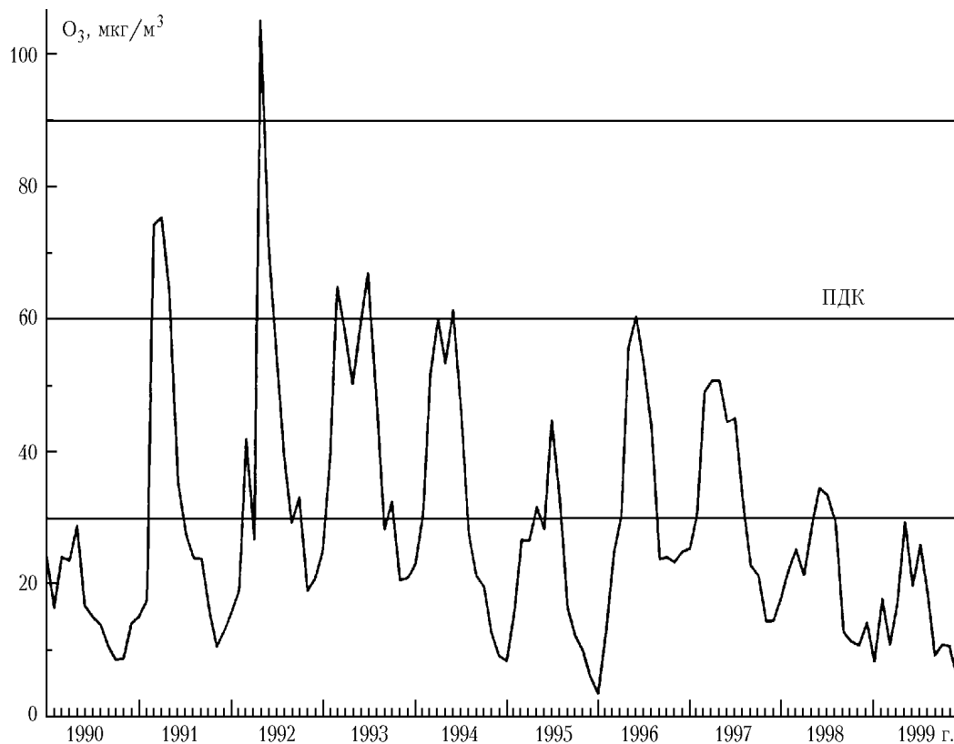
Рис. 6. Среднемесячная концентрация озона в Томске в 1990–1999 гг.
