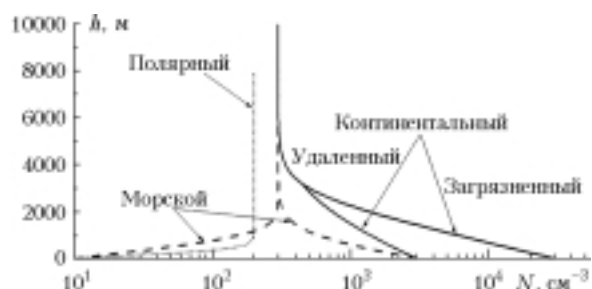
Рис. 1. Характерное вертикальное распределение счетной концентрации аэрозоля [8]
