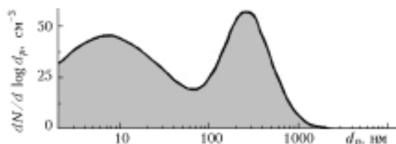
Рис. 2. Характерное распределение аэрозоля по размерам в свободной тропосфере [8]
