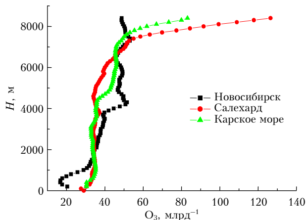
Рис. 12. Вертикальное распределение O 3 над континентом, побережьем и океаном
