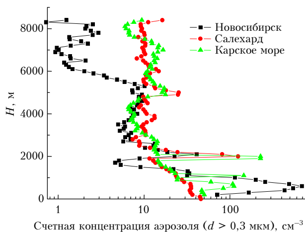
Рис. 13. Вертикальное распределение счетной концентрации аэрозоля над континентом, побережьем и океаном
