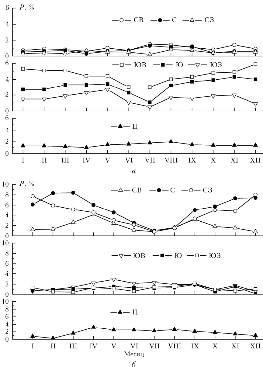
Рис. 3. Повторяемость частей циклона ( a ), антициклона ( б ) в Томске (Ц — центр)
