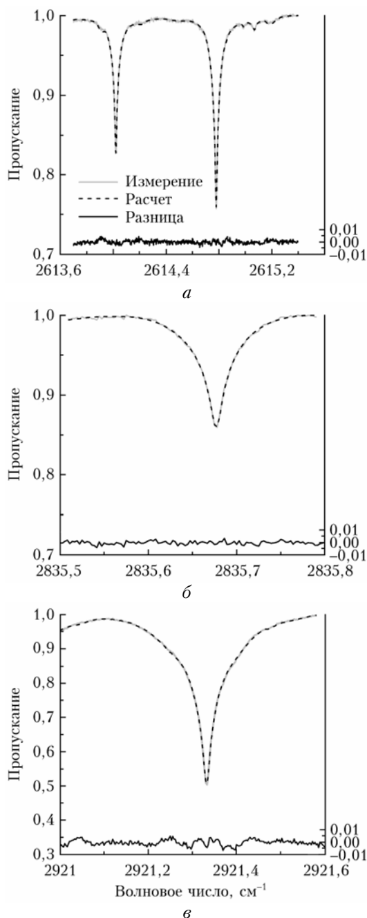
Рис. 3. Результаты подгонки рассчитанного спектра к измеренному 29 мая 2019 г. 08:15:45 UTC для трех микроокон, использующихся при определении ОС CH_4 : а – 2613,70–2615,40 cm^{-1} ; б – 2835,50–2835,80 cm^{-1} ; в – 2921,00–2921,60 cm^{-1}
