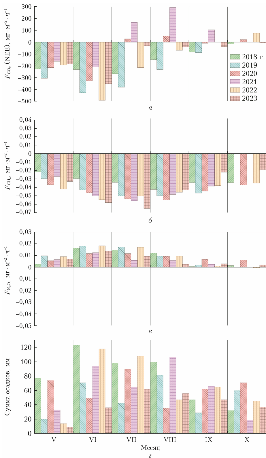
Рис. 6. Среднемесячные удельные потоки парниковых газов, измеренные с помощью прозрачной камеры на участке с растительностью ( a–б ), и месячные суммы осадков ( г )
