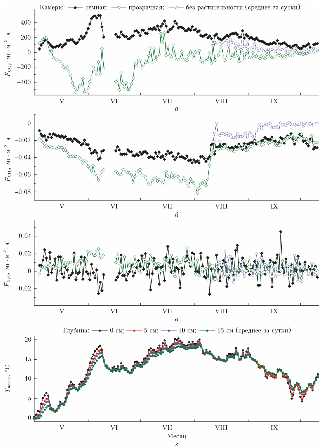
Рис. 2. Среднесуточные значения удельных потоков \text{CO}_2 (а), \text{CH}_4 (б), \text{N}_2\text{O} (в) и температуры почвы (г) в 2023 г.
