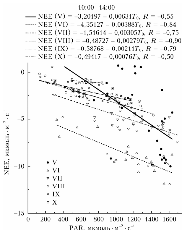
Рис. 8. Зависимость средних дневных (10:00–14:00) значений удельных потоков CO 2 в прозрачной камере с растительностью от среднего дневного значения (10:00–14:00) плотности потока фотосинтетически активной радиации
